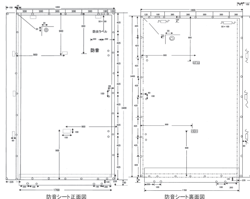
防音シート正面図
